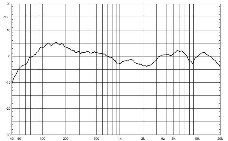
WD15A - preset FOH
