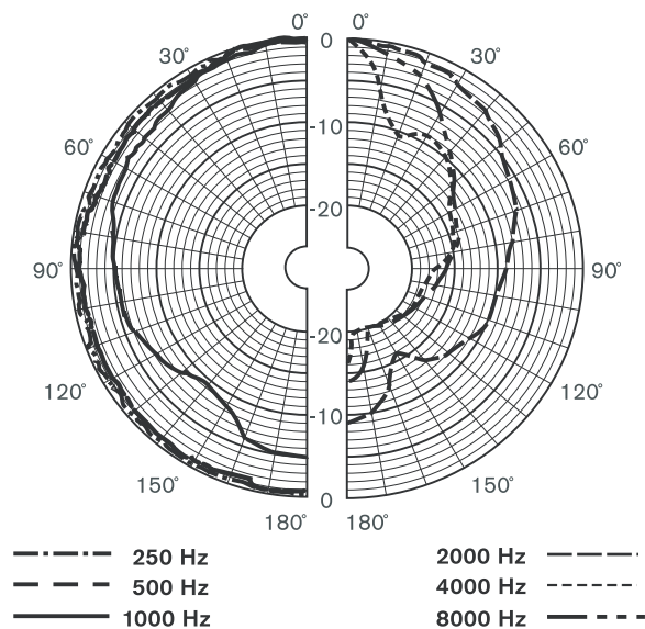
Diagramme polaire (mesuré avec bruit rose)
